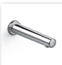
HANSAELECTRA elektronická batéria, DN 15 0088 0010 chróm, Prevádzka na batérie – riadená bezdotykovým elektrickým (infračerveným lúčom), výtok pre nástennú montáž, vyloženie: 225 mm
